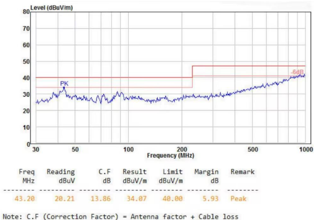
图 6-8 辐射测试垂直方向
