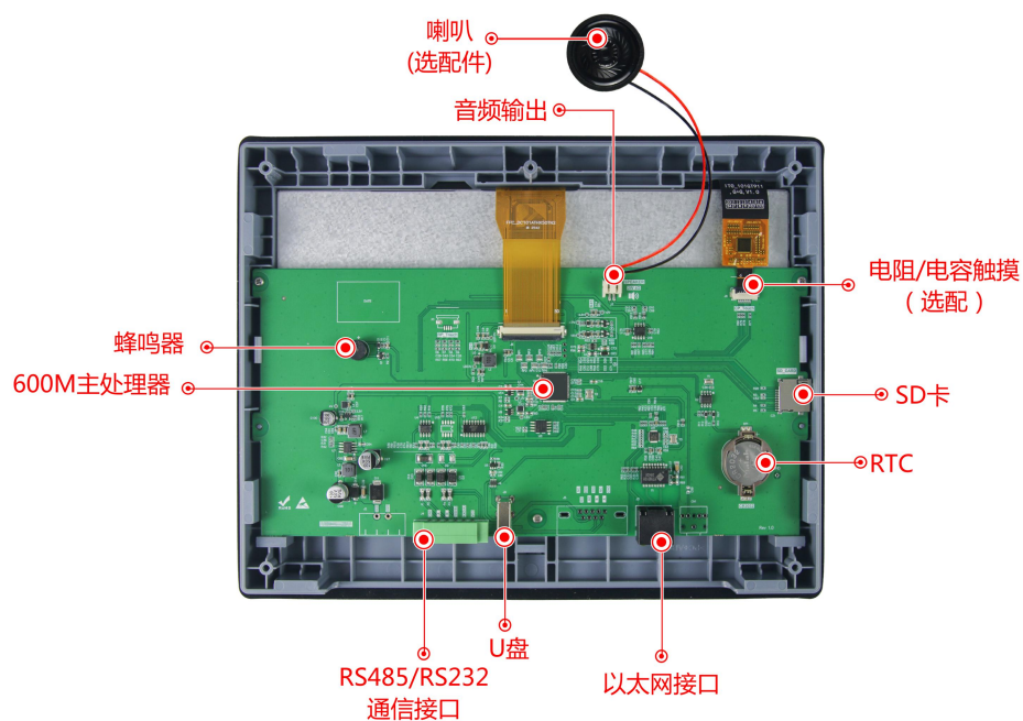
图 1-2 硬件配置图
