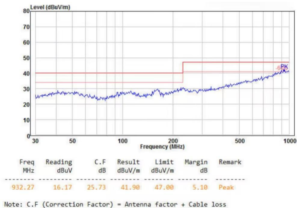
图 6-7 辐射测试水平方向
