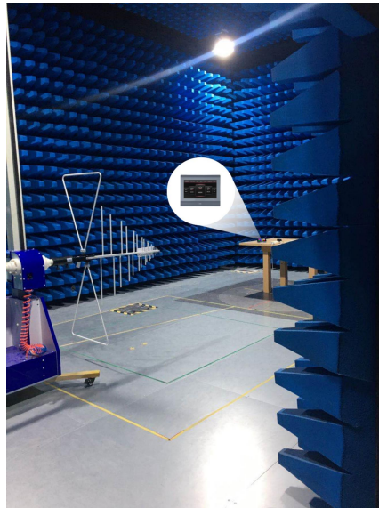
图 6-6 辐射测试图
